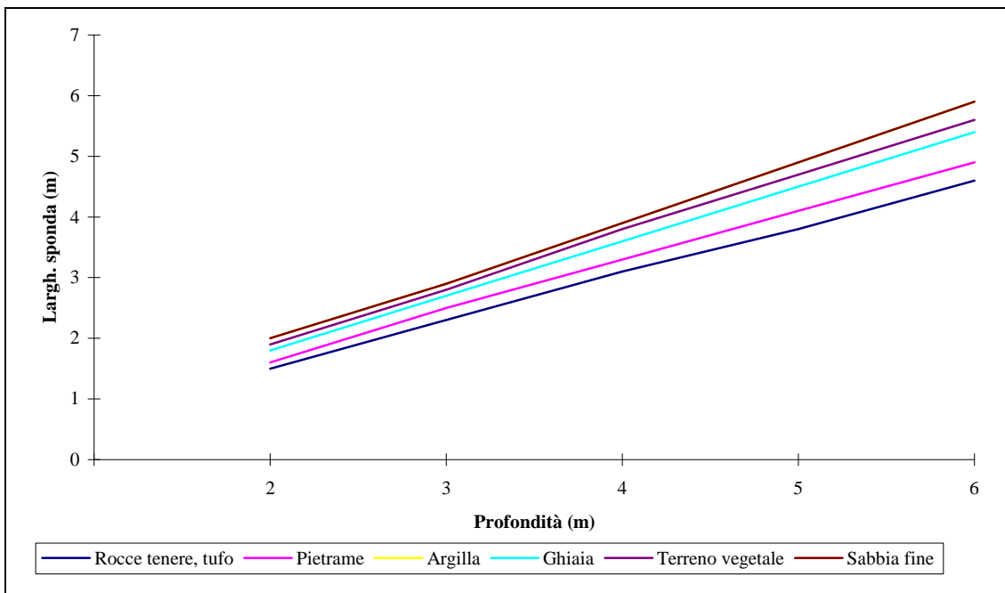
Figura 1 - Stabilità naturale dei pendii asciutti
