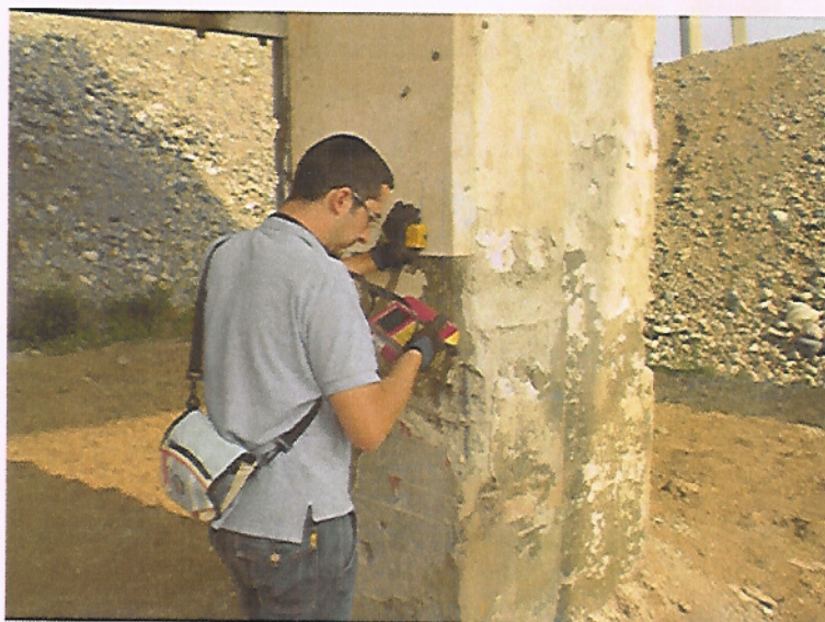
INDAGINE MAGNETOMETRICA
