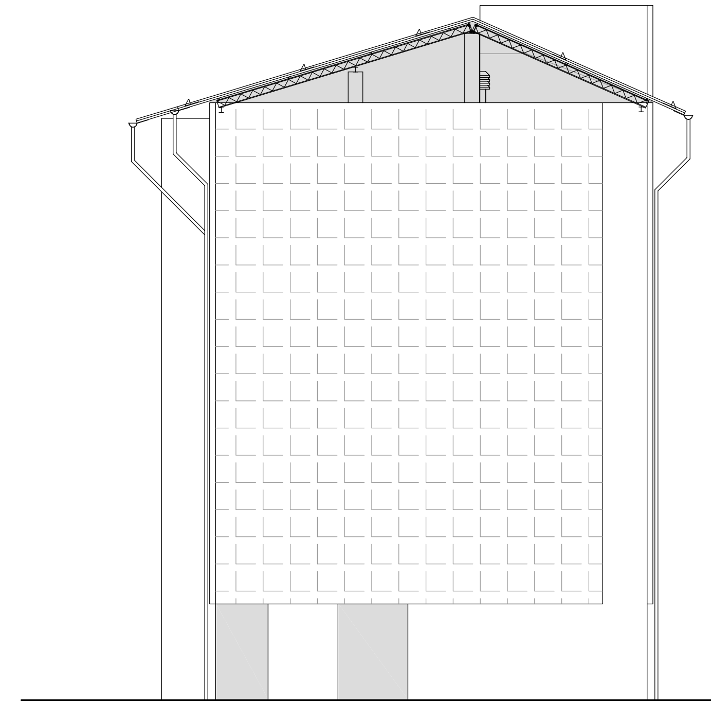
PROSPETTO NORD-EST - FABBRICATO B
