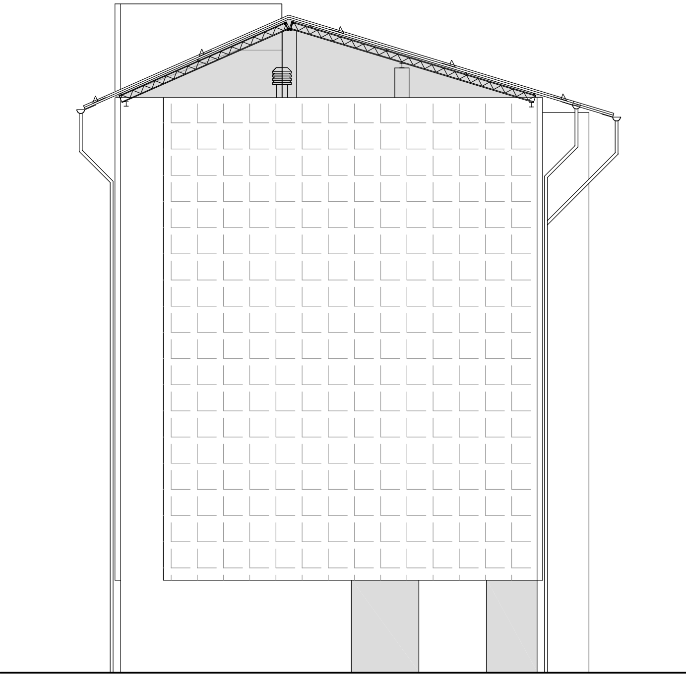
PROSPETTO SUD-OVEST - FABBRICATO B
