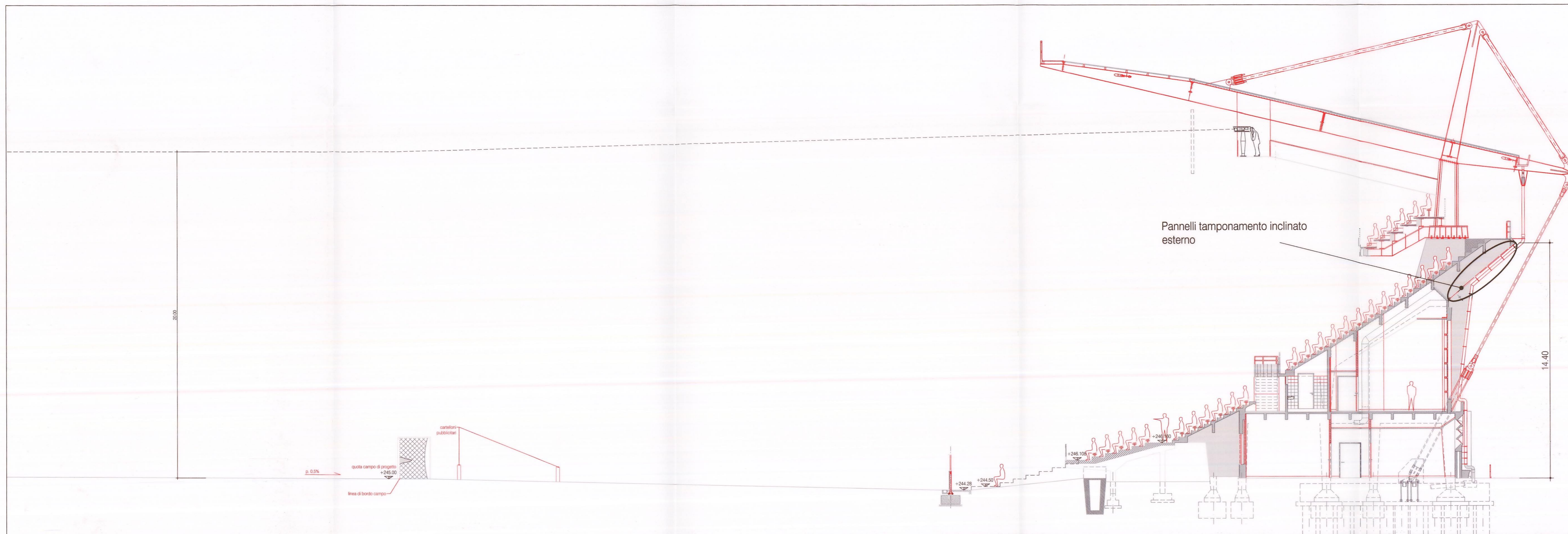
SEZIONE LONGITUDINALE - Y (Curva Nord) - scala 1:100
