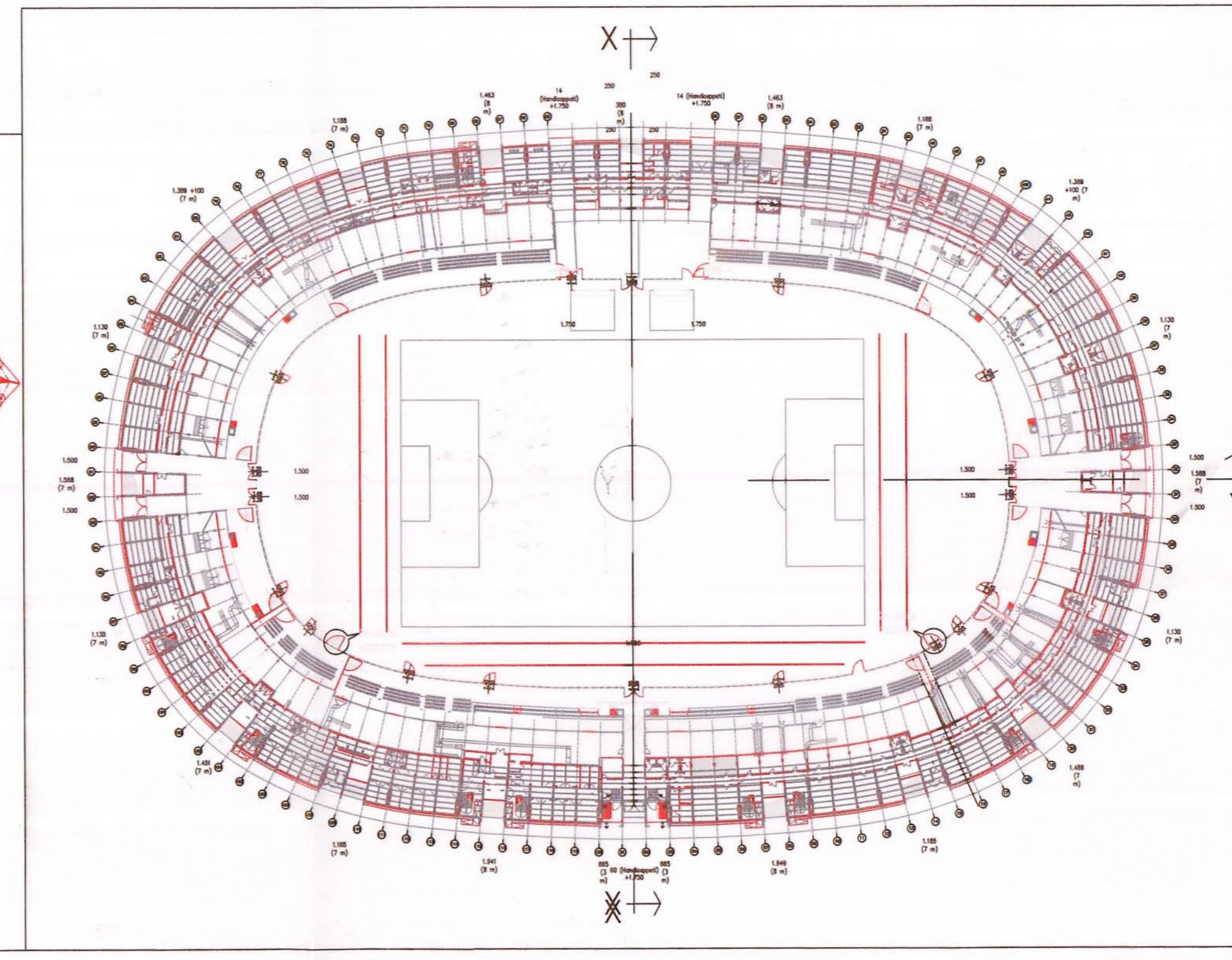
PIANTA COPERTURA - scala 1:1000
