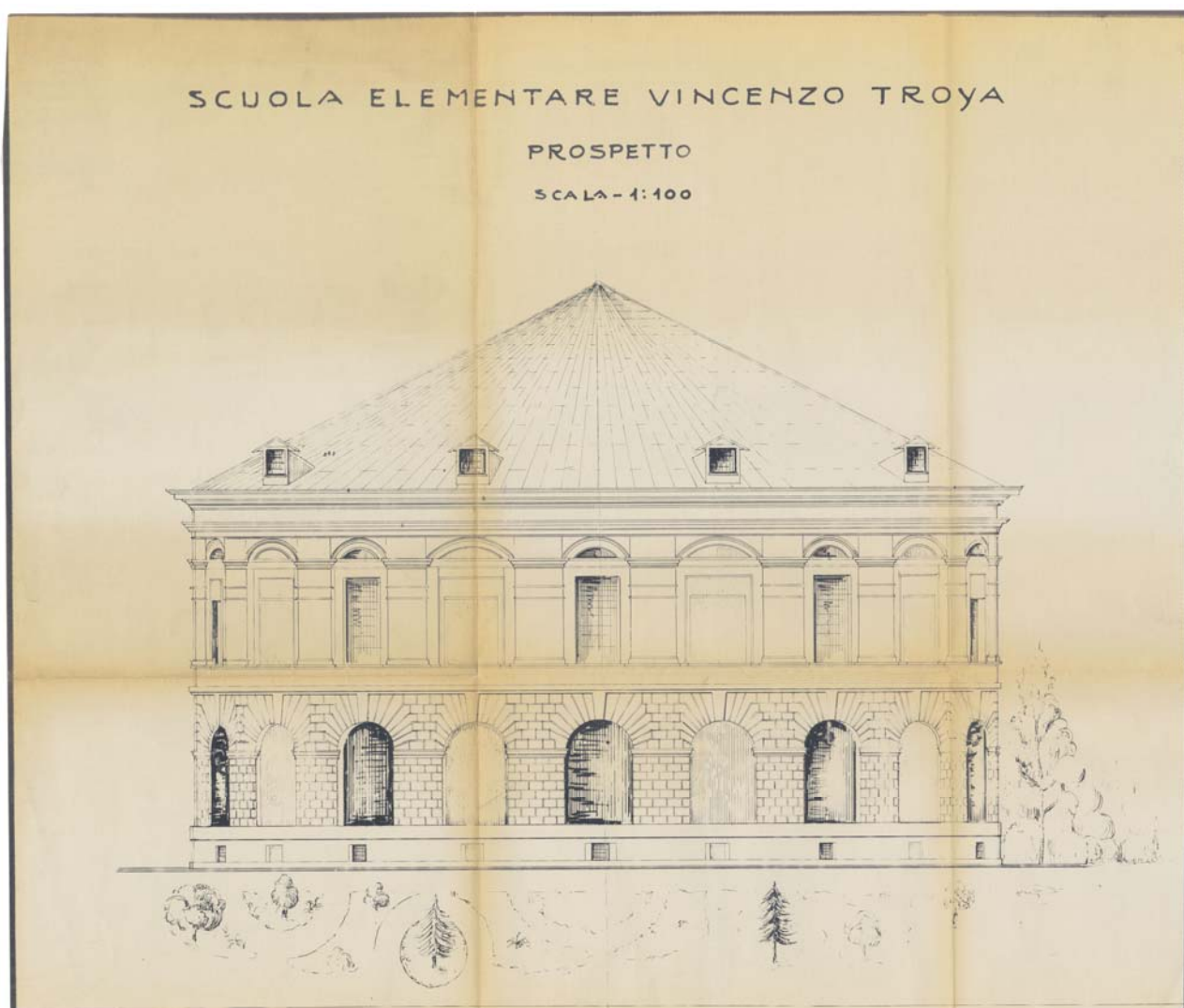
fig. 10) Prospetto della Scuola Elementare Vincenzo Troya , senza data (ASCT, Tipi e disegni , cartella 14, fascicolo 7, n. 21)
