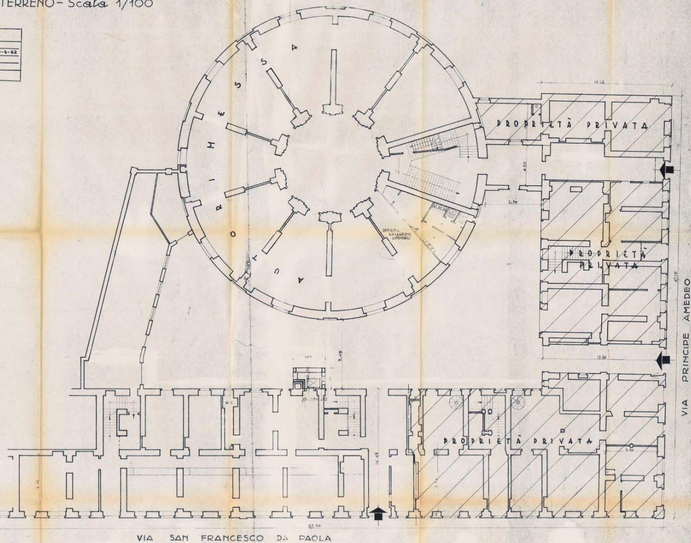
fig. 23) Isolato di San Francesco da Paola, pianta del piano terreno, scala 1:100, 30 .5.1962 (ASCT, Tipi e disegni, cart. 14, fasc. 7 n.. 11)
