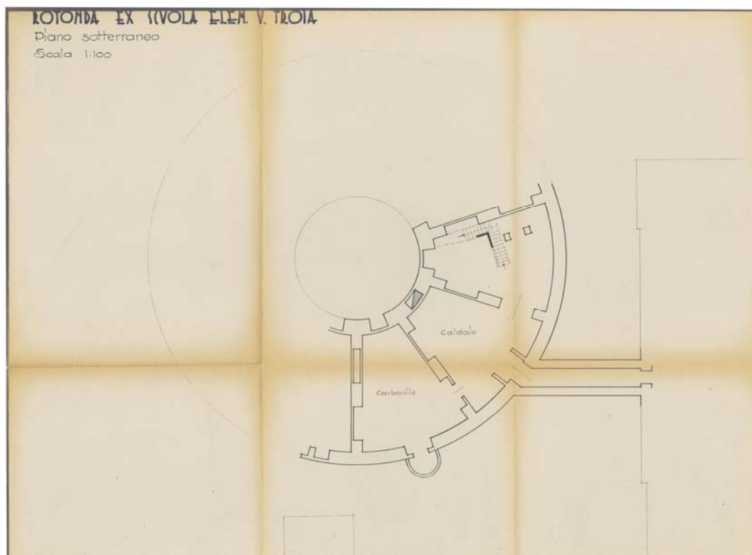
fig. 20 a) Rotonda ex Scuola Elementare V. Troia, pianta piano sotterraneo, scala 1:100, senza data (ASCT, Tipi e disegni , cart. 14, fasc.7, n.17)
