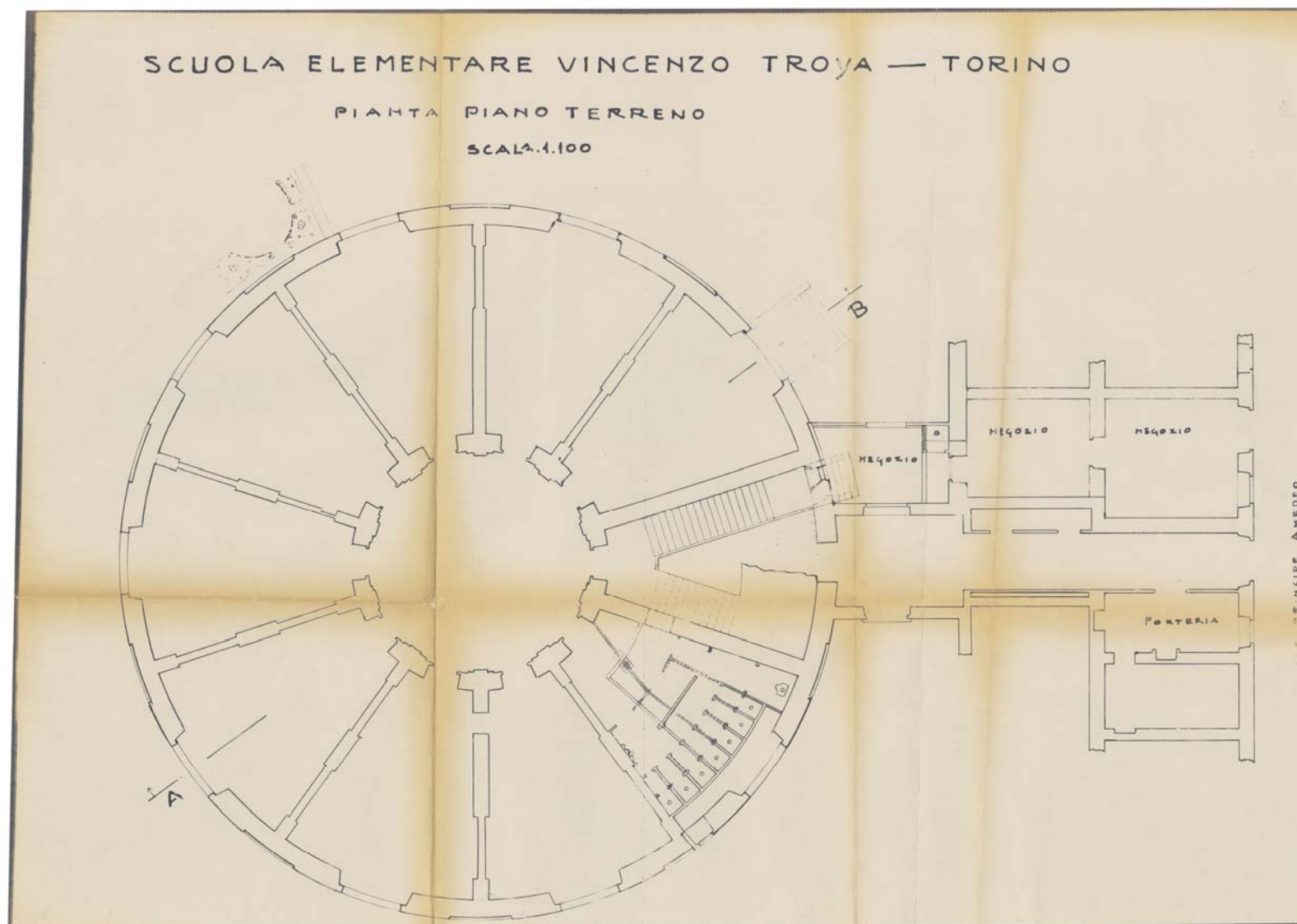
fig. 11) Scuola Elementare Vincenzo Troya, Pianta piano terreno, scala 1:100, senza data (ASCT, Tipi e disegni , cart.14, fasc. 7, n.18)
