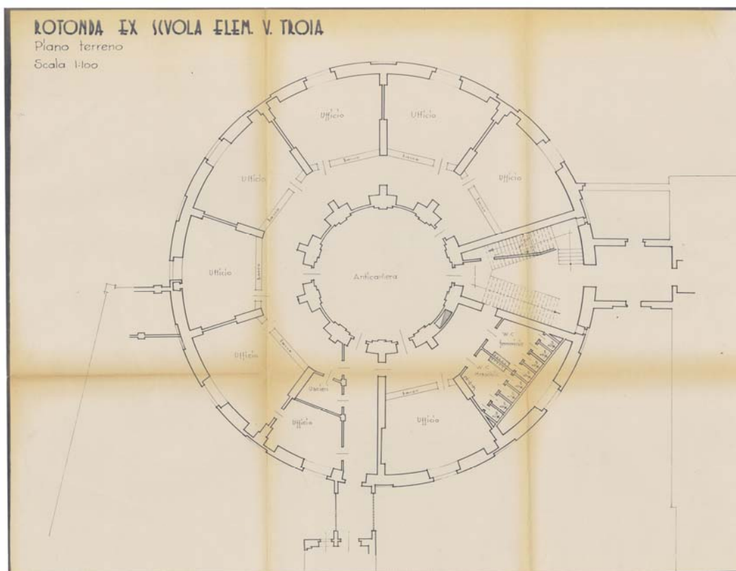
fig. 20 b) Rotonda ex Scuola Elementare V. Troia, pianta piano terreno, scala 1:100, senza data (ASCT, Tipi e disegni , cart. 14, fasc.7, n.18A)
