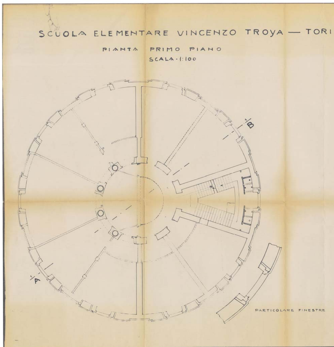
fig. 12) Scuola Elementare Vincenzo Troya, Pianta primo piano, scala 1:100, senza data (ASCT, Tipi e disegni, cart.14, fasc. 7, n.19)
