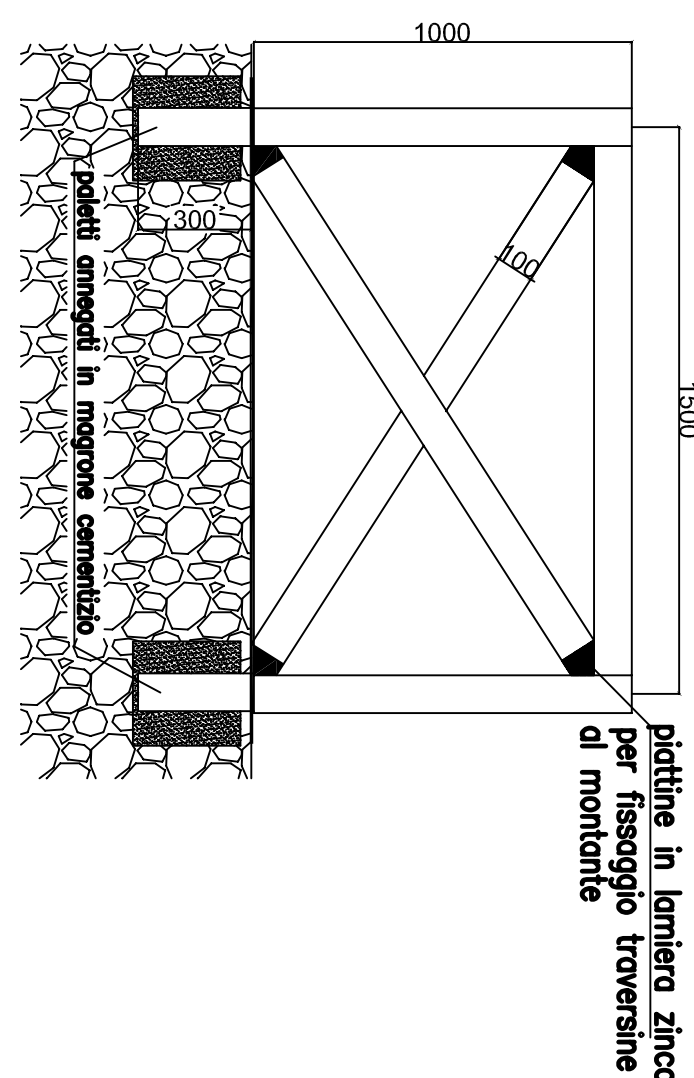
RECINZIONE IN PALETTI LIGNE
