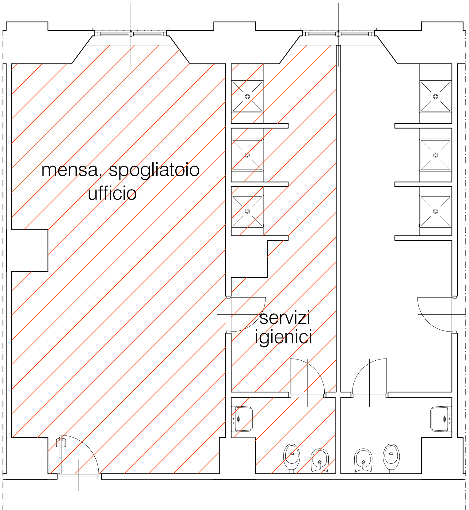
ESTRATTO LOCALI A DISPOSIZIONE PER SERVIZI IGIENICI E SOCIO-SANITARI DEL CANTIERE scala 1:50
