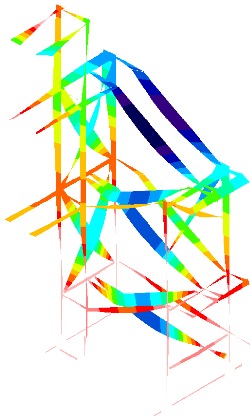
Spostamento verticale per caso di carico n.1 (carichi statici SLU)
