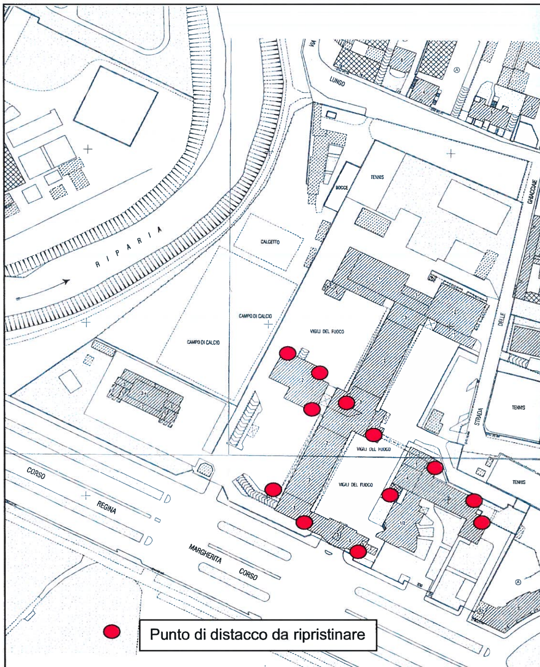
Foto 10 – Intonaci delle facciate ammalorati (mappa dei punti di distacco)
